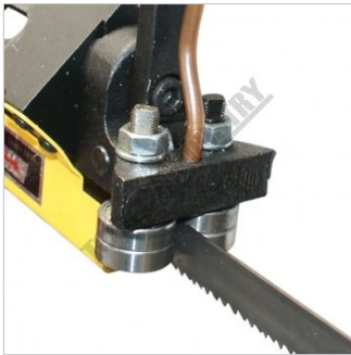
Blade Guide
