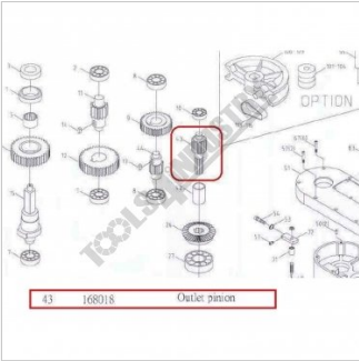
6HX0043 OUTLET PINION 168018
